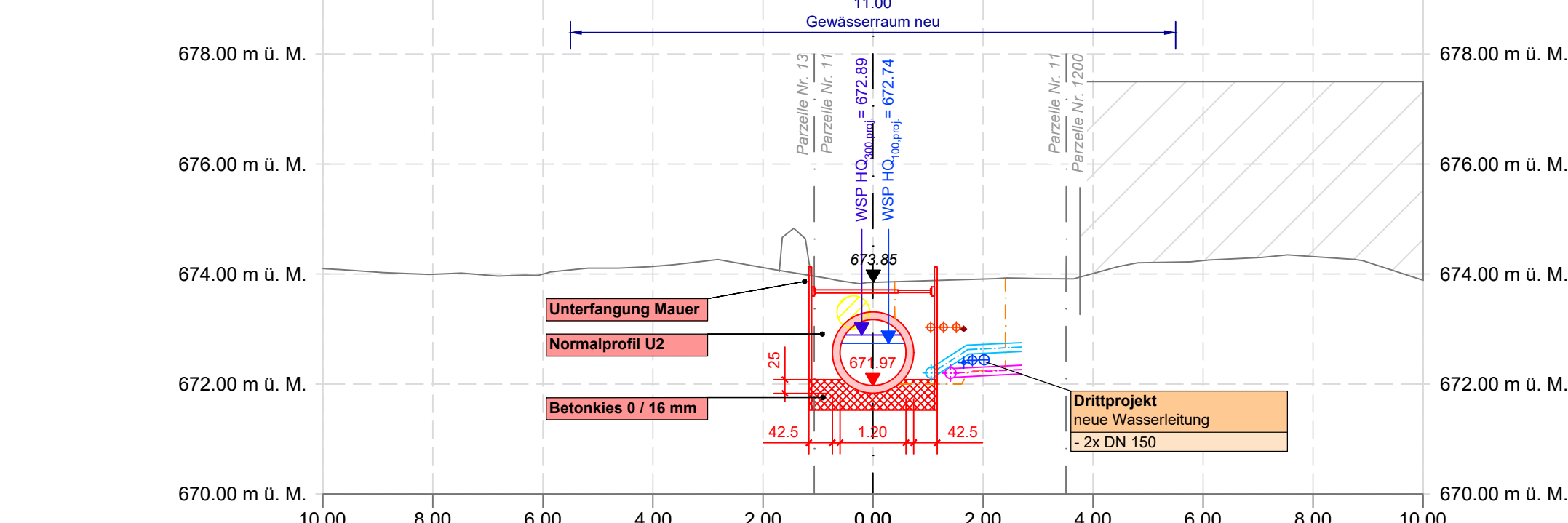
Querschnitt 2.1 1:100
