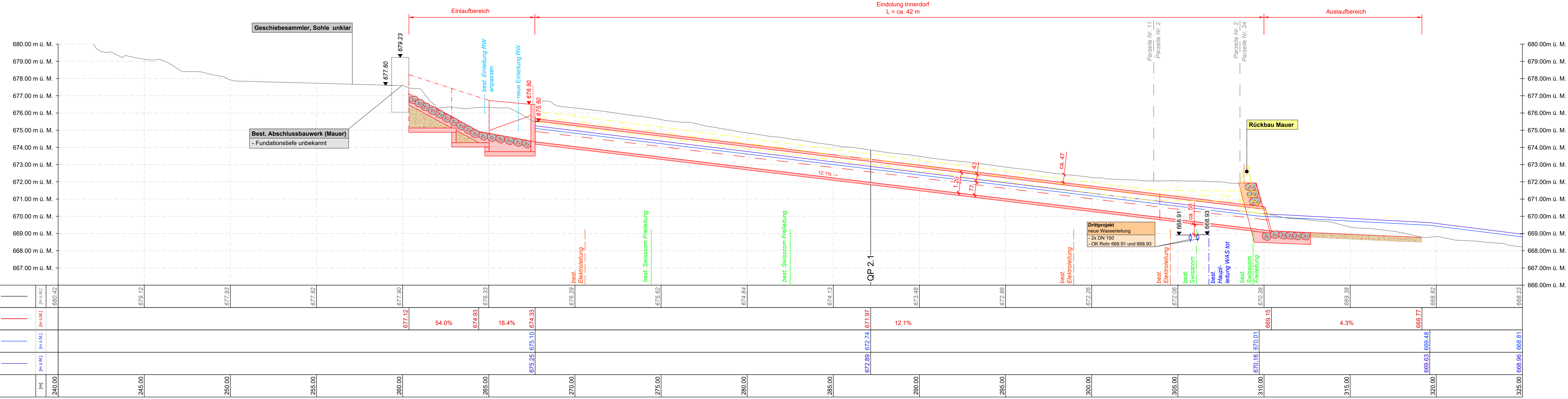
Längenschnitt 1:100
